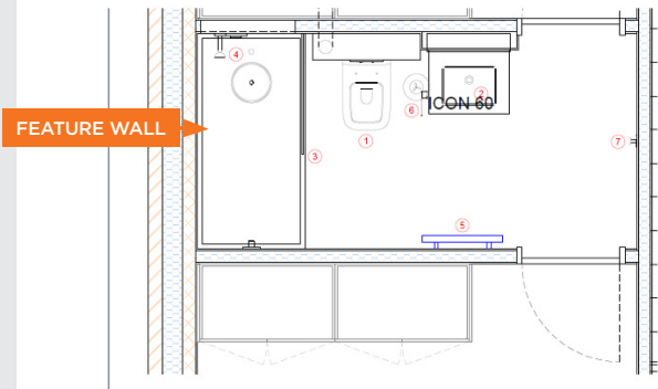
Bedroom 3/4 En Suite
